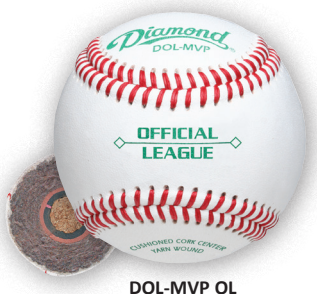
DOL-MVP OL
