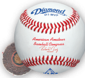
D1-MVP AABC
