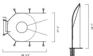
732130 OPTIONAL BARRIER NET SHOWN
